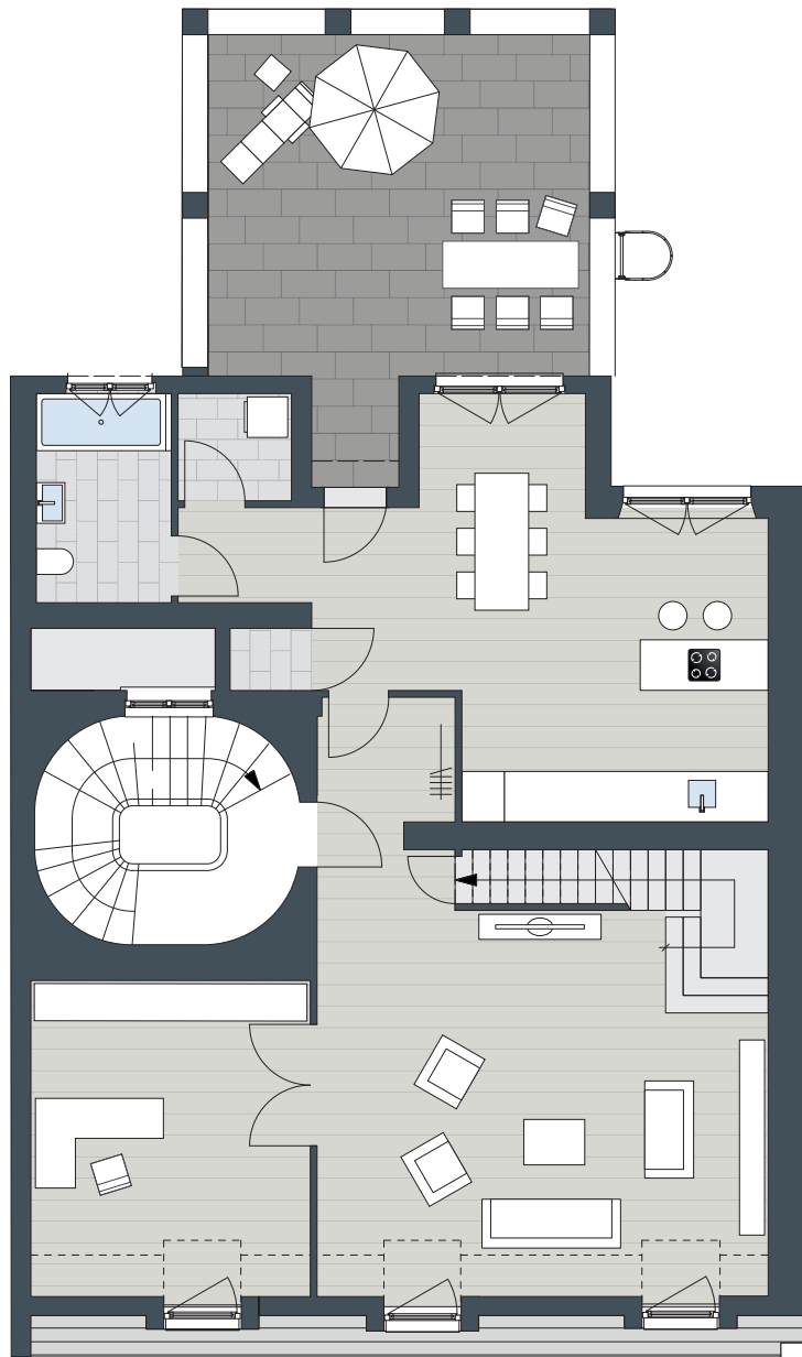
Dachgeschoss
